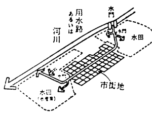
図-3 市街地流通の用水路の基本方式
