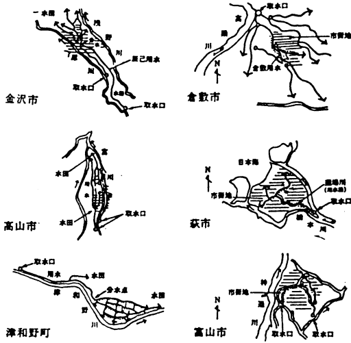
図-3 市街地流通の用水路の基本方式
