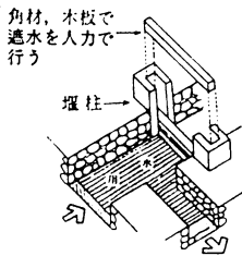
図-2 角落式の基本型
